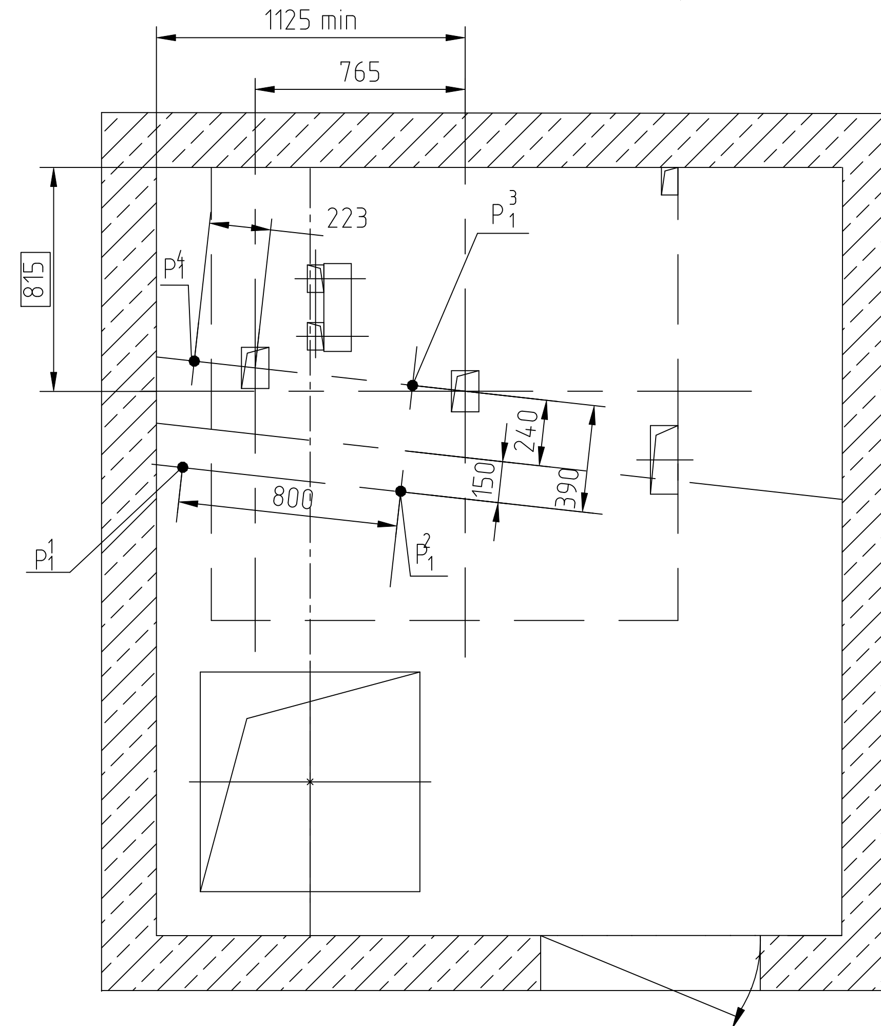
В-В(1) 1:20 Рис.2 остальное см. рис.1
